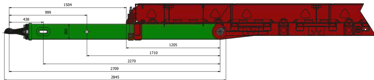
A-A (1 : 10)
